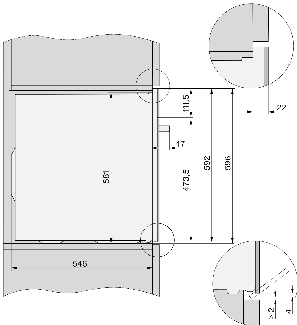
Вид сбоку
